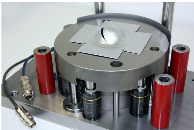
Abb. 1 In der Prüfmaschine drückt ein halbkugelförmiger Stempel das Werkstück bis zu einer definierten Tiefe ein. Die Analyse des Kraft-Weg-Verlaufs erlaubt detaillierte Rückschlüsse auf die Qualität des Materials.
