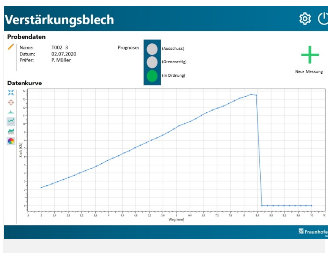
Abb. 2 Mithilfe von Machine-Learning-Algorithmen analysiert die Software die Daten aus zahlreichen Messpunkten und beurteilt die Eignung des Blechs für den Fertigungsprozess. Das Ampelsymbol zeigt das Ergebnis: »Ausschuss«, »grenzwertig« oder »in Ordnung«.
